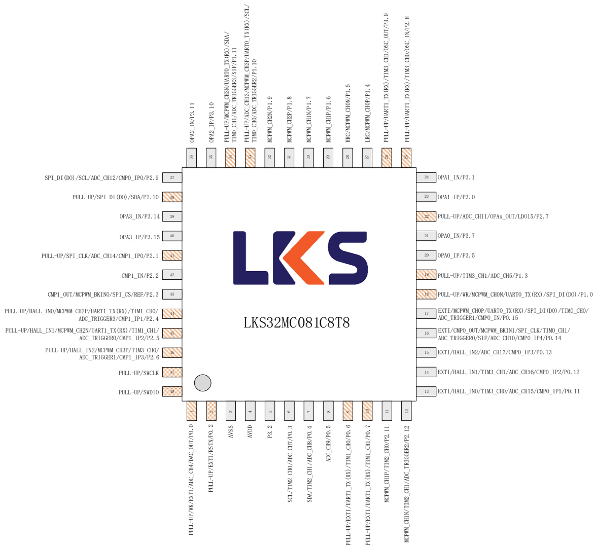
图 3-2 LKS32MC081C8T8(B)/LKS32MC088C6T8(B)管脚分布图
